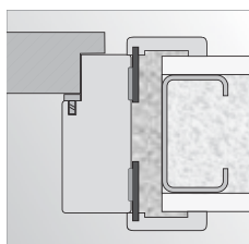
montáž do pěny do stěny ze sádkartonové desky
