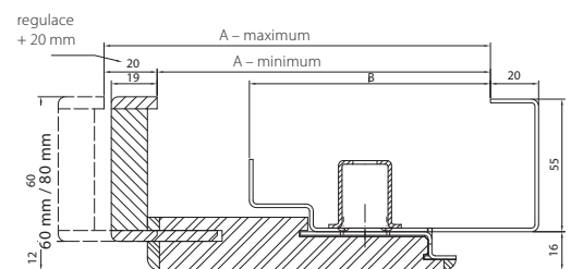
průřez zárubně PROJEKT Premium
