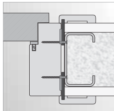
montáž na vruty do stěny ze sádkartonové desky
